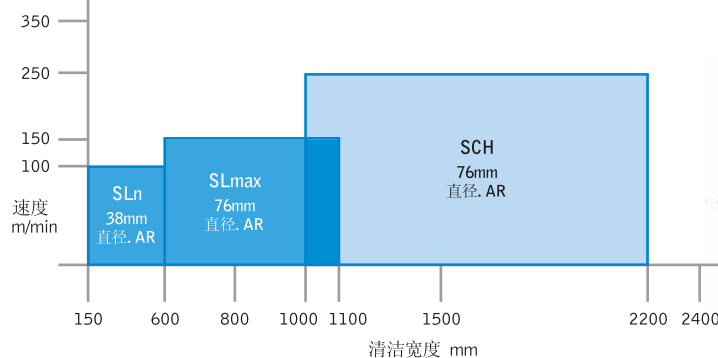
SLn / SLmax / SCH 产品图 无护罩，无滑轨
